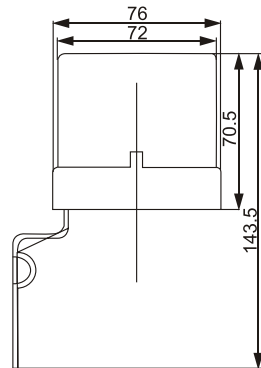
Exterior dimension(mm)
