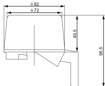
Exterior dimension(mm)
